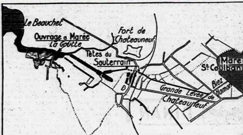
Schéma d'un plan de dénoisement des marais de Châteauneuf par la Rance.
